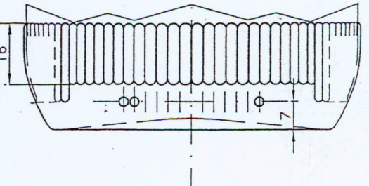
Sect.B-B N.90 FLUTES N.90 COSTE
